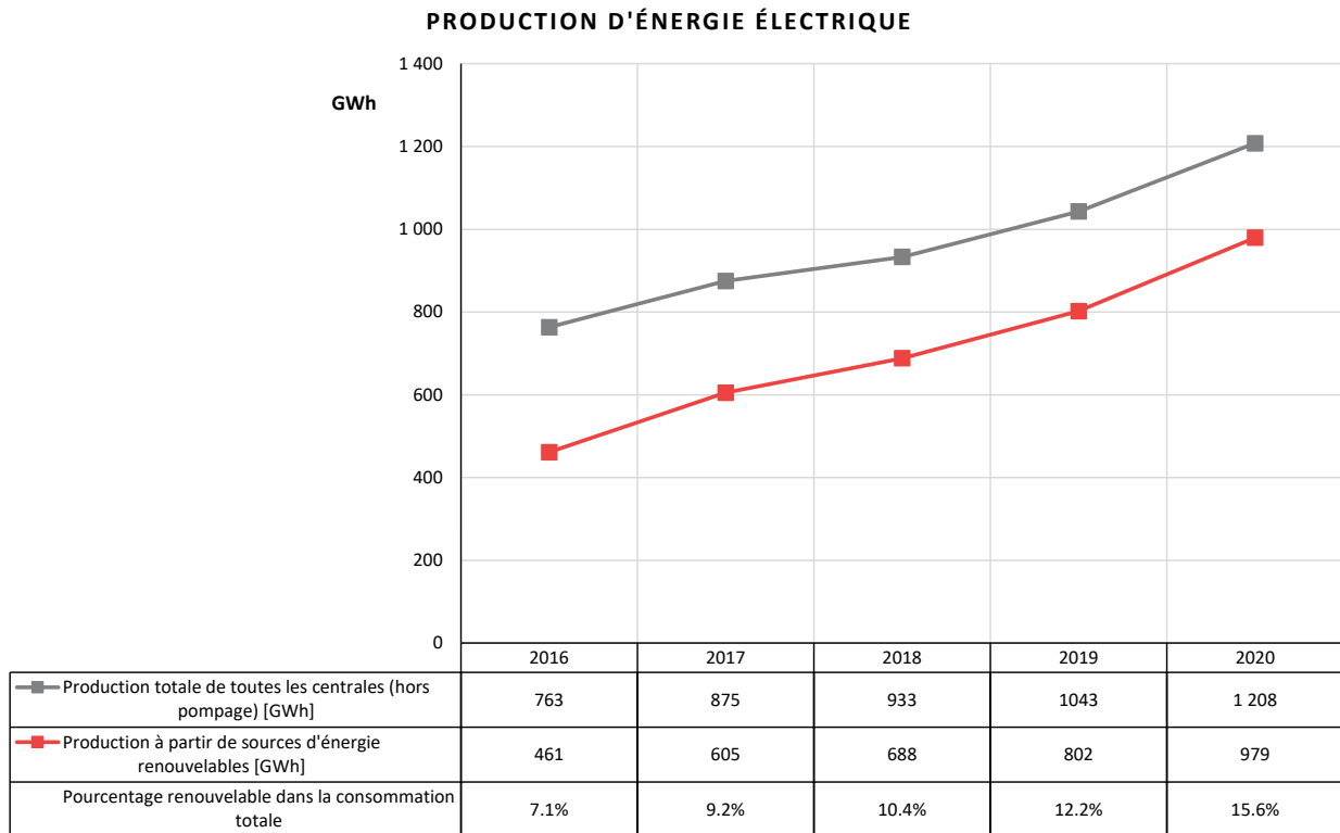
GRAPHIQUE 4 – PRODUCTION TOTALE D'ÉLECTRICITÉ ET PRODUCTION D'ÉLECTRICITÉ À PARTIR DE SOURCES RENOUVELABLES
