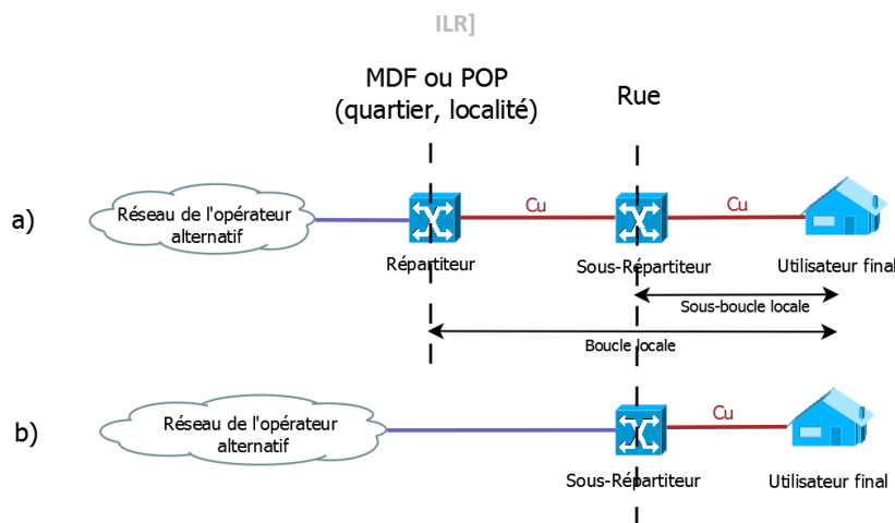
Graphique 2-1: Illustration des prestations de dégroupage de la boucle et de la sous-boucle locale de la paire de cuivre [Source:
